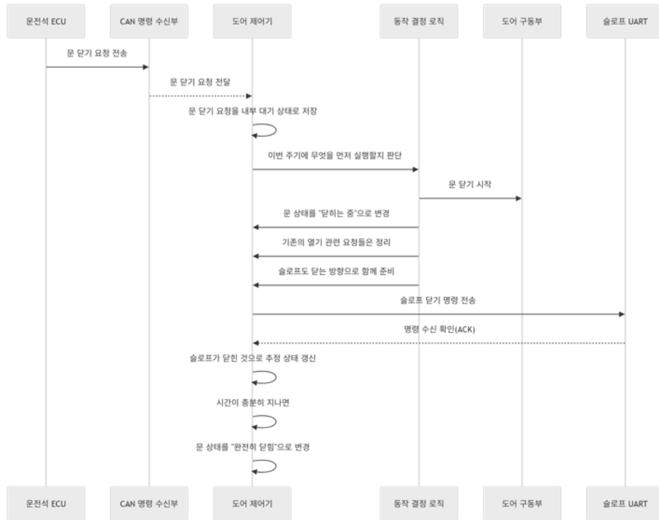
운전석 ECU에서 문 및 slope 닫힘 명령 수신 시
