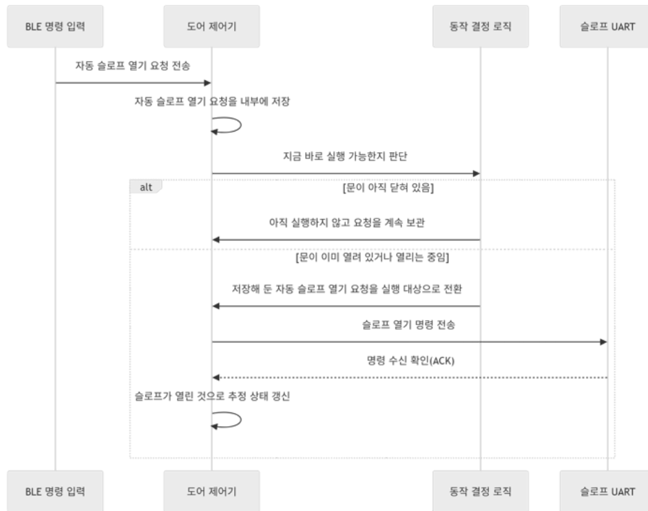
BLE 처리 구조
