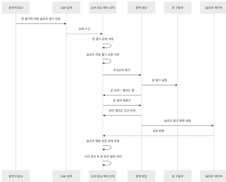
운전석 ECU에서 문 및 슬로프 열림 명령 수신 시
